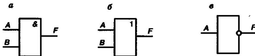
Рис. 1.5. Логические элементы
